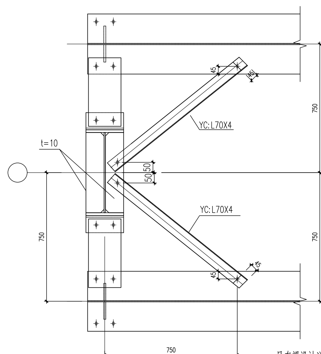
DCL—*中间柱中跨安装节点
