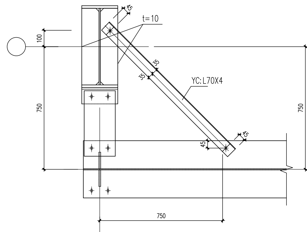
DCL—*端部安装节点
